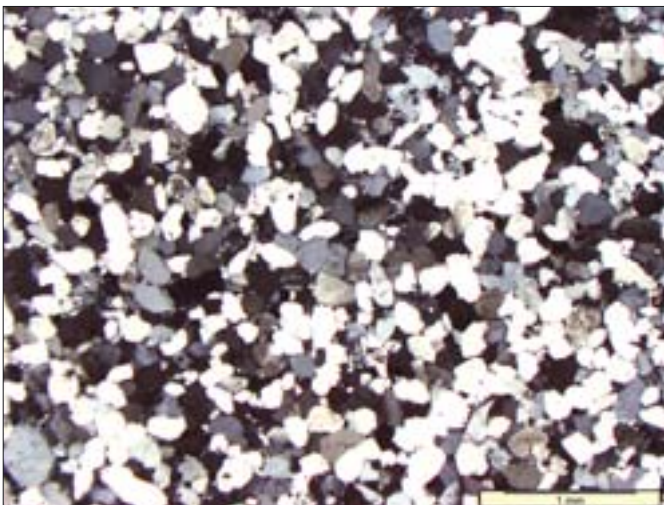
12. Obraz mikroskopowy fragmentu próbki trzonu kolumny z aniołem (dep. 564) uzyskany w świetle przechodzącym przy skrzyżowanych nikolach.
