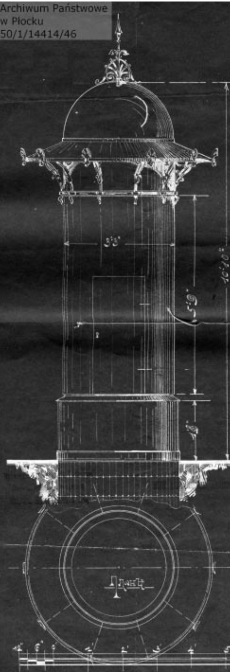
Projekt słupa ogłoszeniowego załączony do kontraktu
