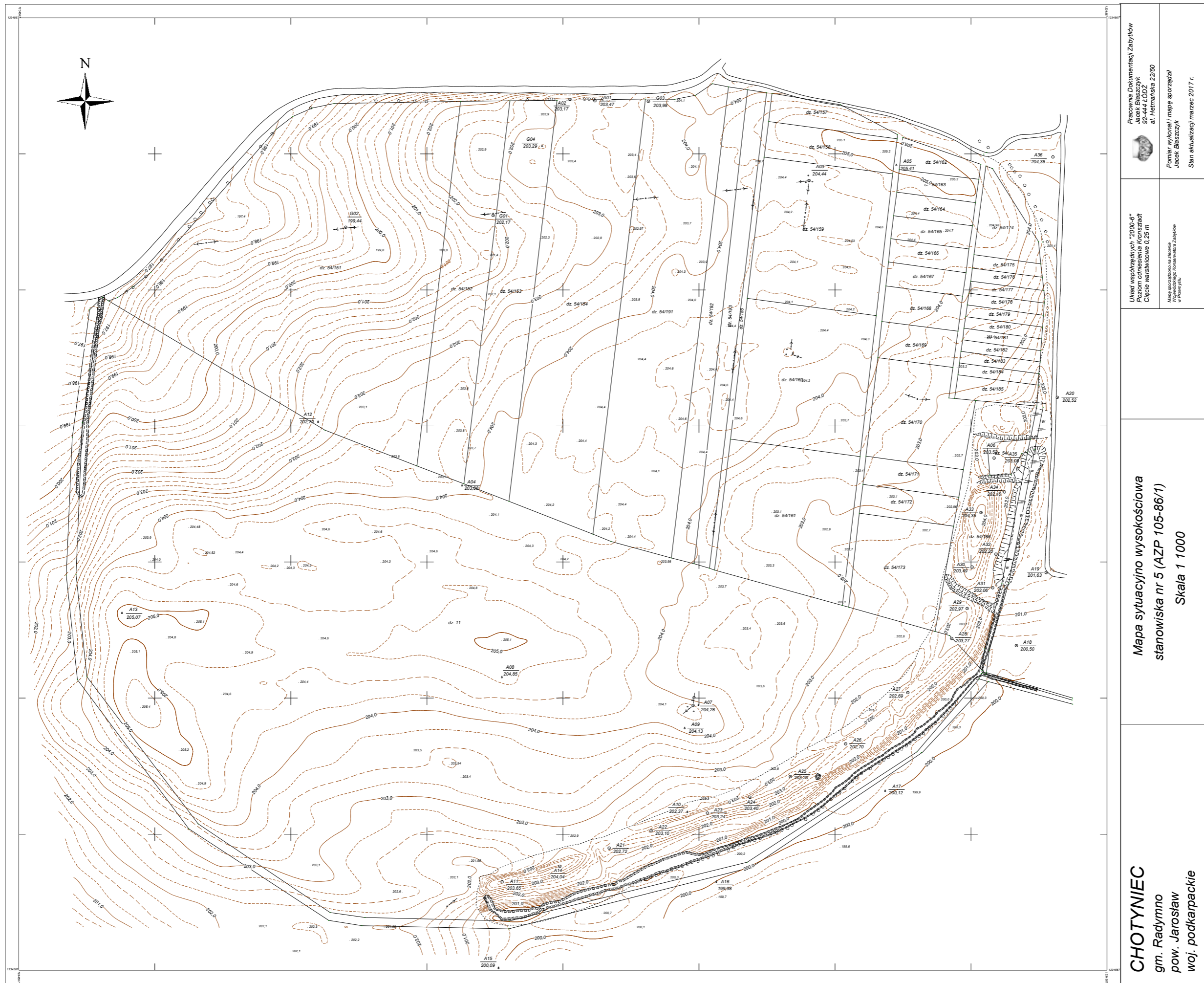
Ryc. 2. Chotyńiec, pow. jarosławski, stan. 1. Plan sytuacyjno-wysokościowy (wykonany przez J. Błaszczyka na podstawie pomiarów 2016–2017)
