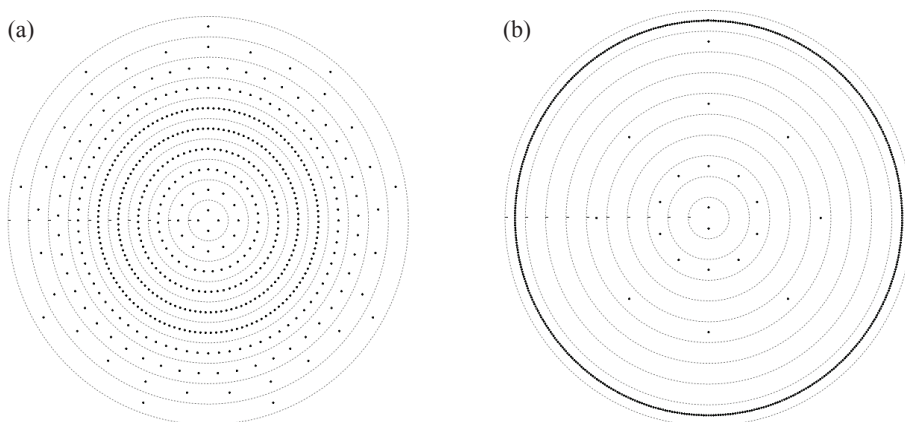
Rys. 7. Wykres koncentryczny (a) centralności bliskości i (b) centralności wektora własnego dla przedsiębiorstw w największym komponencie
