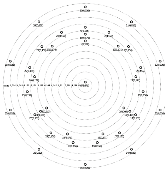
Rys. 3. Wykres koncentryczny hipotetycznej sieci (w nawiasie wynik centralności wektora własnego)
