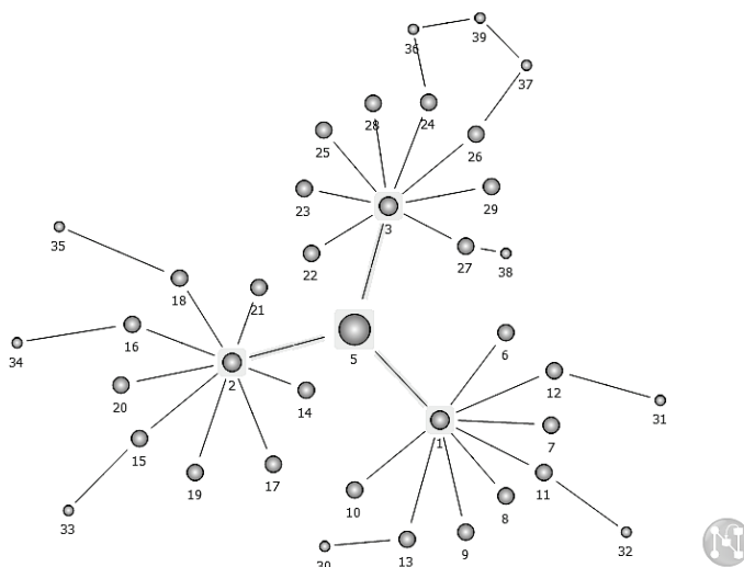
Rys. 2. Hipotetyczna sieć z trzema centrami (węzły 1, 2, 3) i jednym łącznikiem (węzeł 5) – wielkość powierzchni poszczególnych węzłów jest proporcjonalna do centralności wektora własnego
