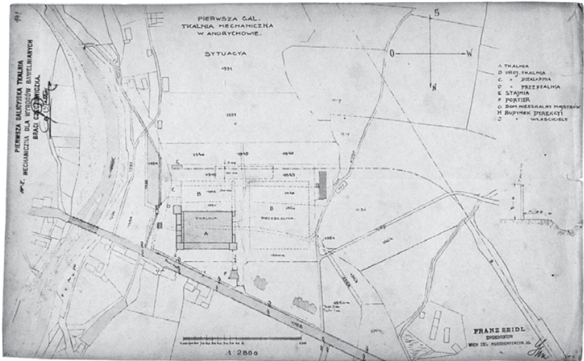
Plan sytuacyjny w podziałce 1:2880, będący załącznikiem do wniosku o pozwolenie na budowę. Podziałka 1:2880 była powszechnie stosowana na austriackich mapach katastralnych (APB-B sygn. akt 13/493/8, s. 141)
