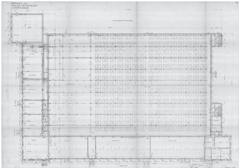
Projekt hali tkalni, będący załącznikiem do wniosku o pozwolenie na budowę. Na rysunku zaznaczono przebieg wałów transmisyjnych, przenoszących napęd od maszyny parowej do poszczególnych krosien (APB-B, MA 13/493/8, s. 145)
