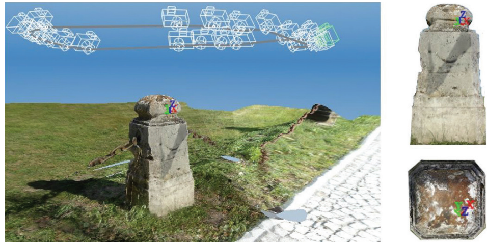
II. 3. Słupek ogrodzenia, model 3D oraz widoki płaskie (oprac. L. Smirnowa)
