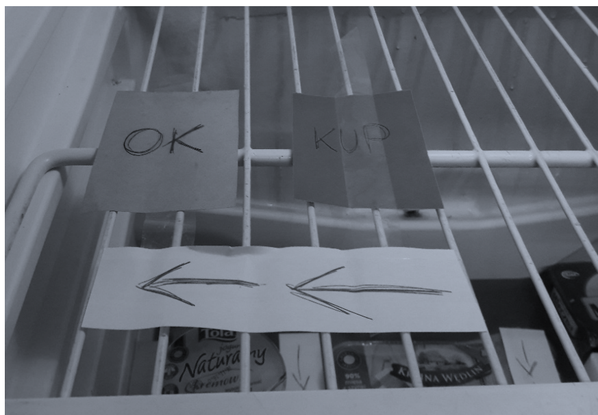
Rysunek 7. System kanban do zarządzania zapasem kartonów z mlekiem
