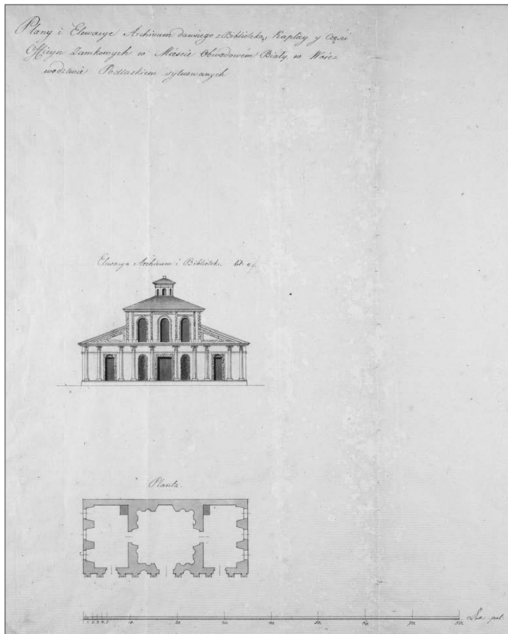
Elewacja i rzut poziomy budynku archiwum i biblioteki zamkowej w Białej, autorstwa S. Kozłowskiego (ok. 1830). AGAD, Zbiór kartografii, 9-2, arkusz 3; fot. Karol Zgliński.
