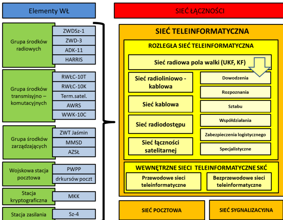
Rys. 4. Elementy składowe sieci łączności budowane w ramach Węzła Łączności
