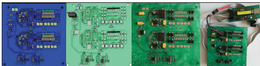
Rys. 3. Sterownik silników krokowych: a) projekt PCB; b) projekt 3D; c) gotowy układ; d) programowanie układu
