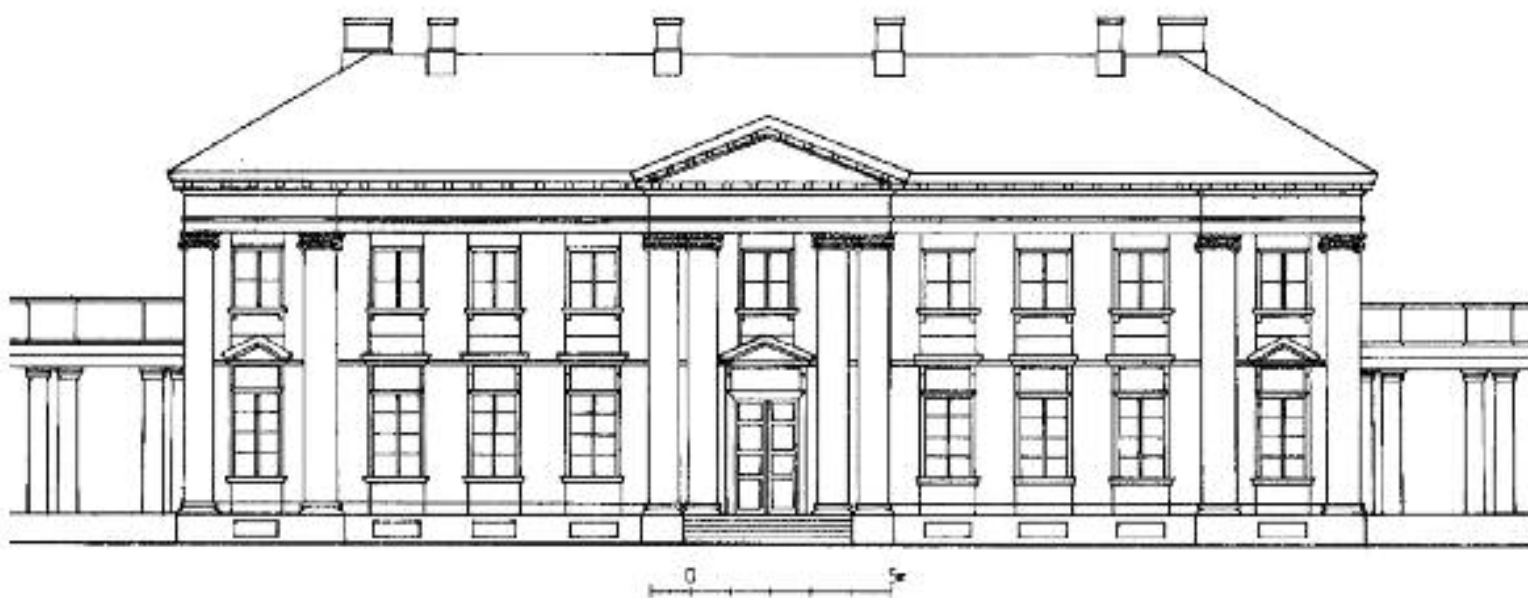
15. Elewacja frontowa pałacu. Rys. M. Skarżyńska-Wawrykiewicz, 2004 r. 15. Front elevation of the palace. Drawing: M. Skarżyńska-Wawrykiewicz, 2004.
