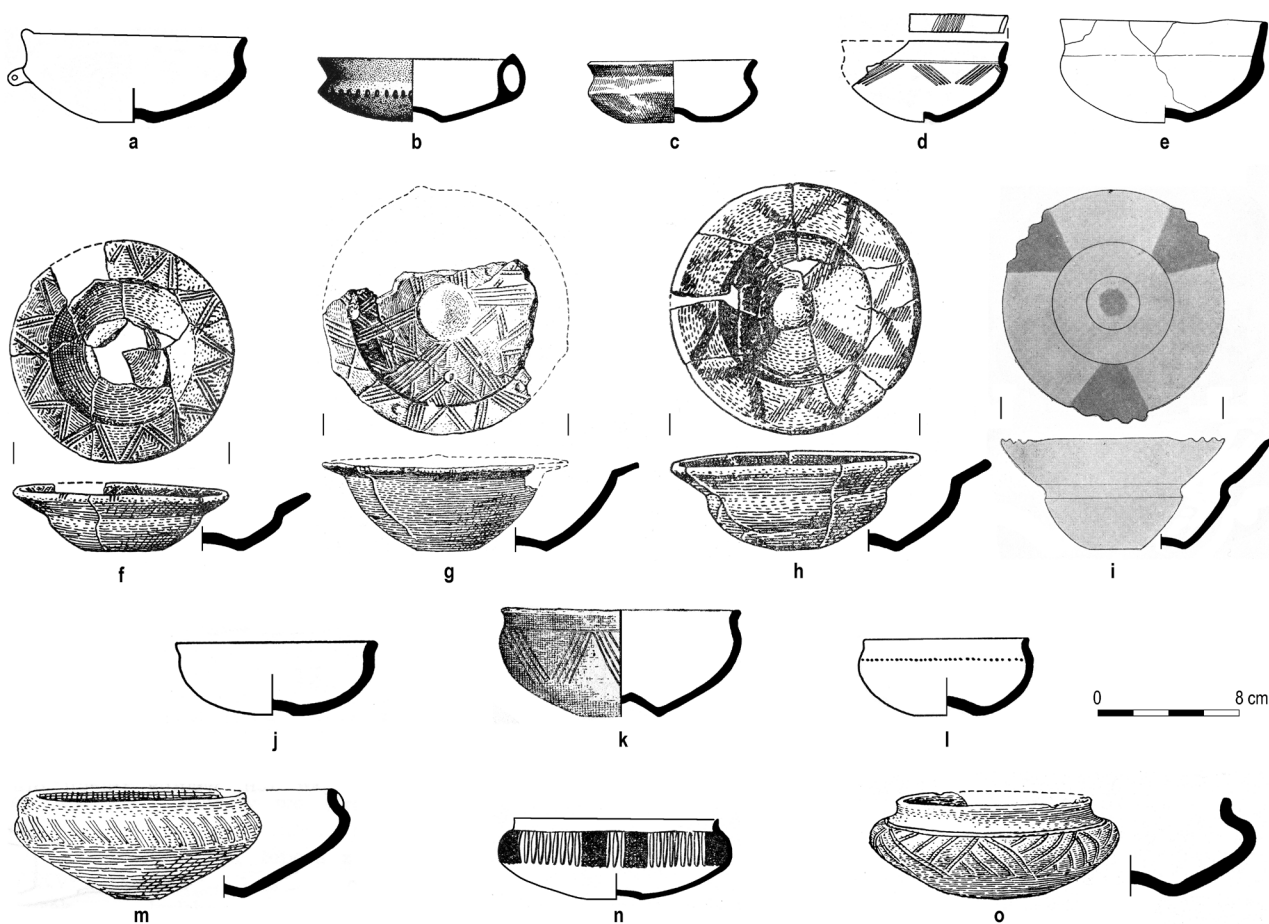
Ryc. 10. Miseczki typu II/C (a–c) oraz podtypów II/D 1 (d, e) i II/D 2 (f–i) z omfalosami 1/a, typu II/E z omfalosami 1/a (j, l) i 1/c (k) oraz typu II/F z wariantu 1/a (m–o).
