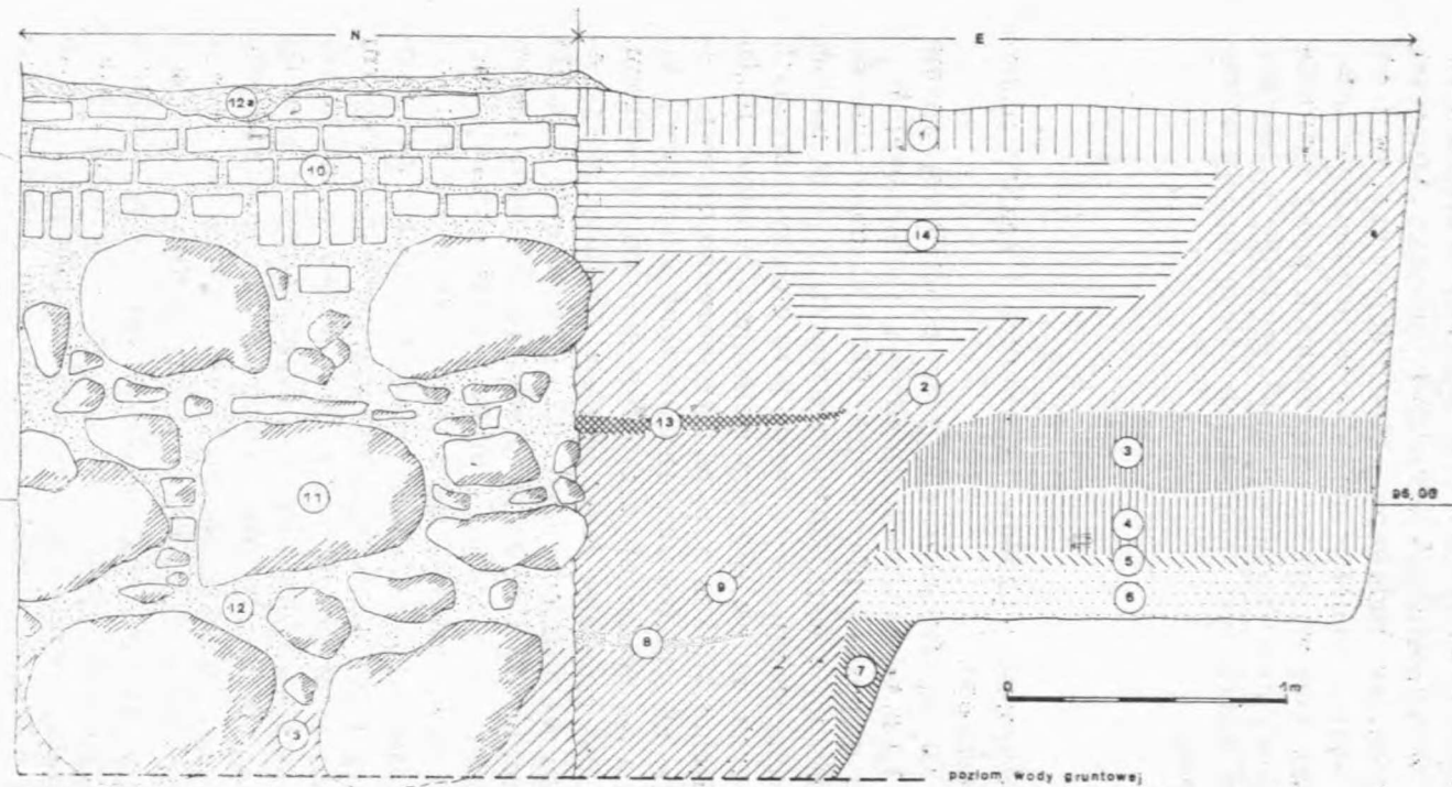
Rys. 4. Wykop I, profil północny i wschodni (nr 1 na rys. 1)
