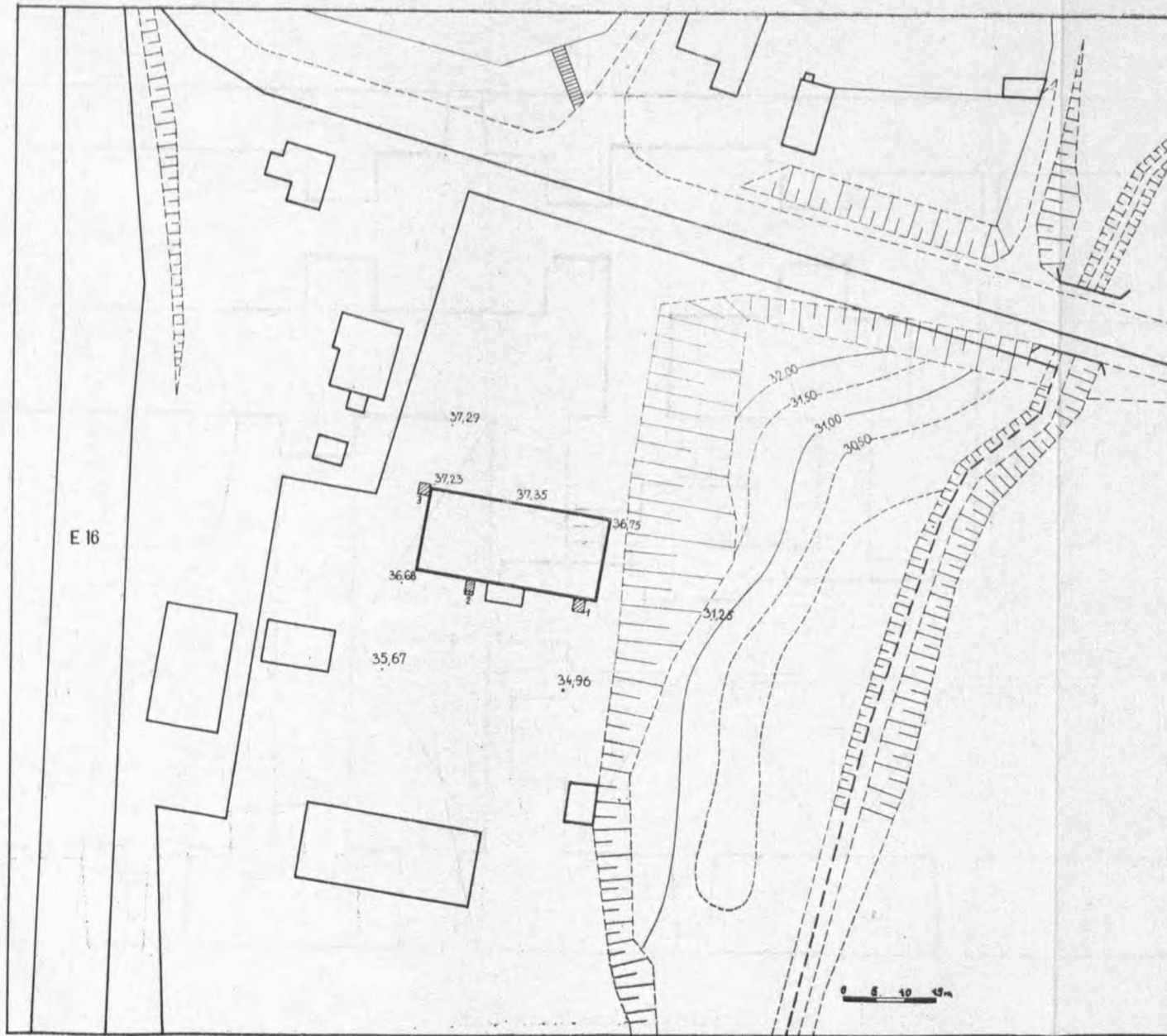
Rys. 1. Plan sytuacyjny z naniesionymi wykopami
