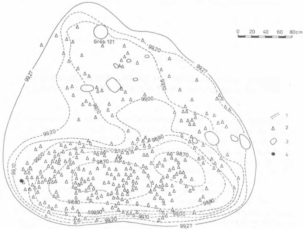
Rys. 1. Wilkowice, gm. Wartkowiec, stan. 1. Plan chałupy nr 13
