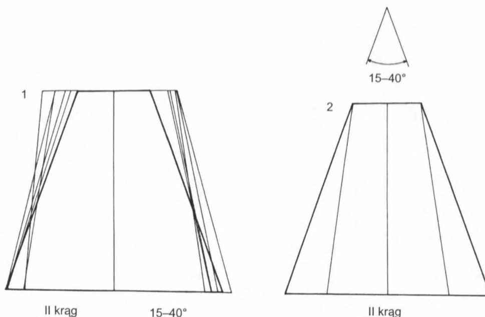
Ryc. 7. Krąg 2. 1 – schemat zbieżności bocznych ścianek stel; 2 – zbioreczy układ bocznych ścianek stel; 15–40° – oznaczony kąt zbieżności ścianek Abb. 7. Steinkreis 2. 1 – Konvergenzschemata der Seitenwände; 2 – Sammelanordnung der Seitenwände; 15–40° – Konvergenzwinkel der Wände
