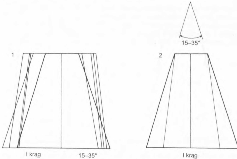
Ryc. 3. Krağ 1. 1 – schemat zbieżności bocznych ścianek stel; 2 – zbiorczy układ bocznych ścianek stel; 15–35° – oznaczony kąt zbieżności ścianek Abb. 3. Steinkreis 1. 1 – Konvergenzschema der Seitenwände; 2 – Sammelanordnung der Seitenwände; 15–35° – Konvergenzwinkel der Wände
