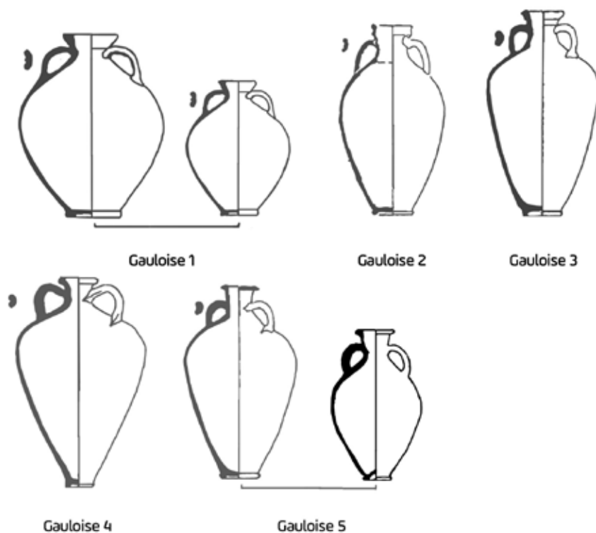
Ryc. 1. Amfory galijskie typu Gauloise 1, Gauloise 2, Gauloise 3, Gauloise 4, Gauloise 5 (F. Laubenheimer, Vins, huiles et sauces, Paris 1990, s. 166).
