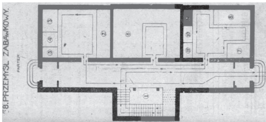
Ilustracja 1. Plan parteru budynku wystawowego ( Powszechna Wystawa Krajowa, Poznań. Katalog Główny, obejmuje przemysł, samorządy, wychowanie fizyczne i instytucje kulturalno-oświatowe, Poznań 1929, s. 268 )
