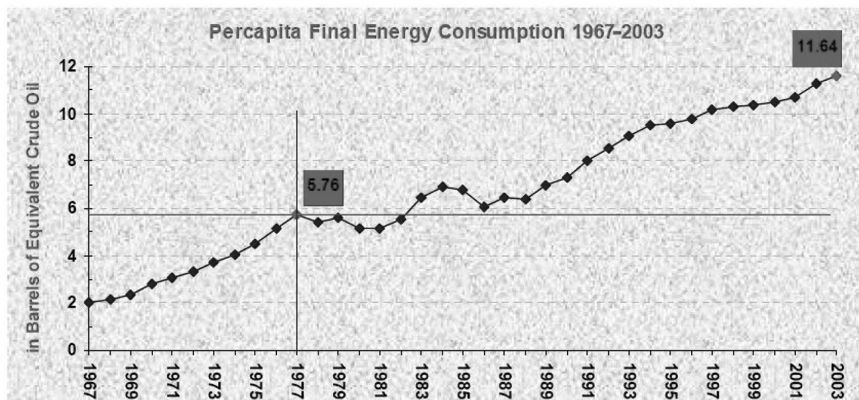
Wykres 2. Wzrost konsumpcji energii w Iranie. Lata 1967–2003
