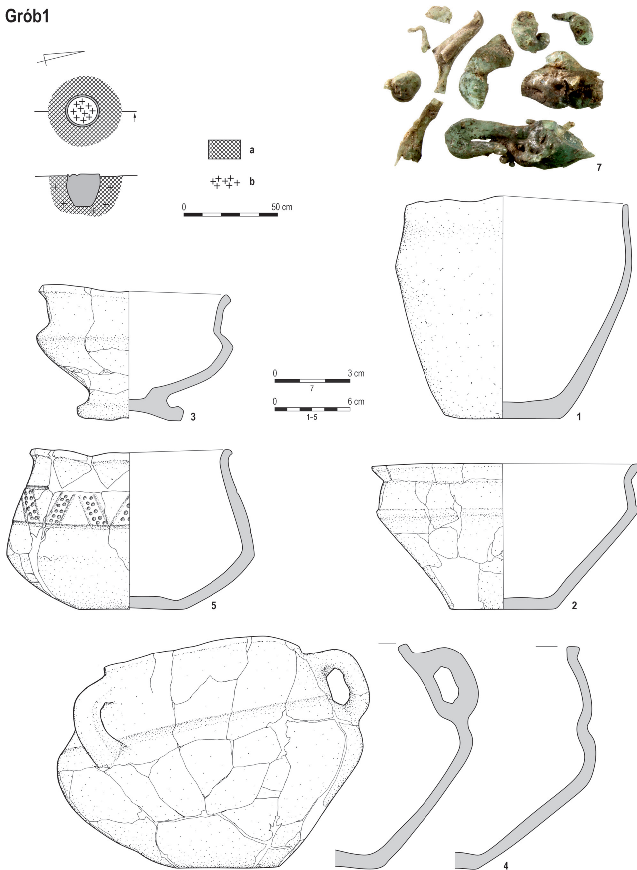
Ryc. 6. Kurki, pow. działdowski, stan. III. Obiekt 1: a – czarna ziemia; b – przepalone kości; 1–5 – glina; 7 – szkło.
