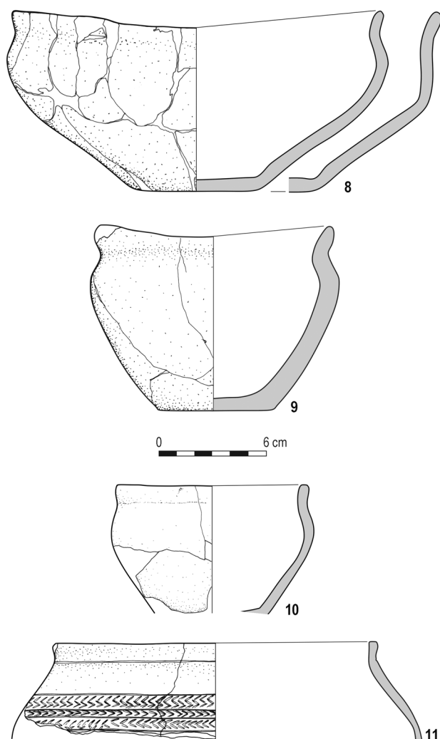
Ryc. 8. Kurki, pow. działdowski, stan. III. Obiekt 2. 8–11 – glina. Rys.: A. Czubińska
