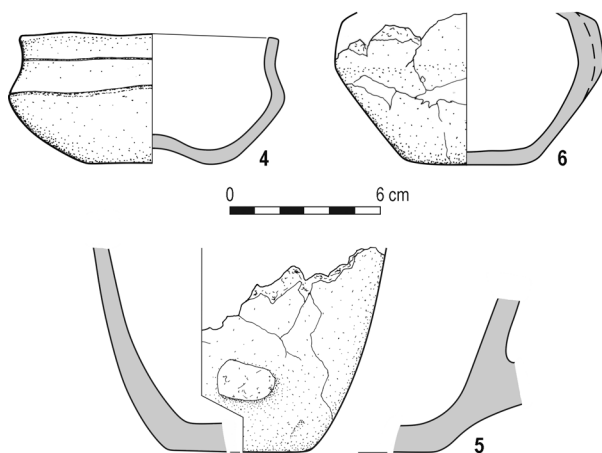
Ryc. 11. Kurki, pow. działdowski, stan. III. Obiekt 23. 8–11 – glina. Rys.: A. Czubińska
