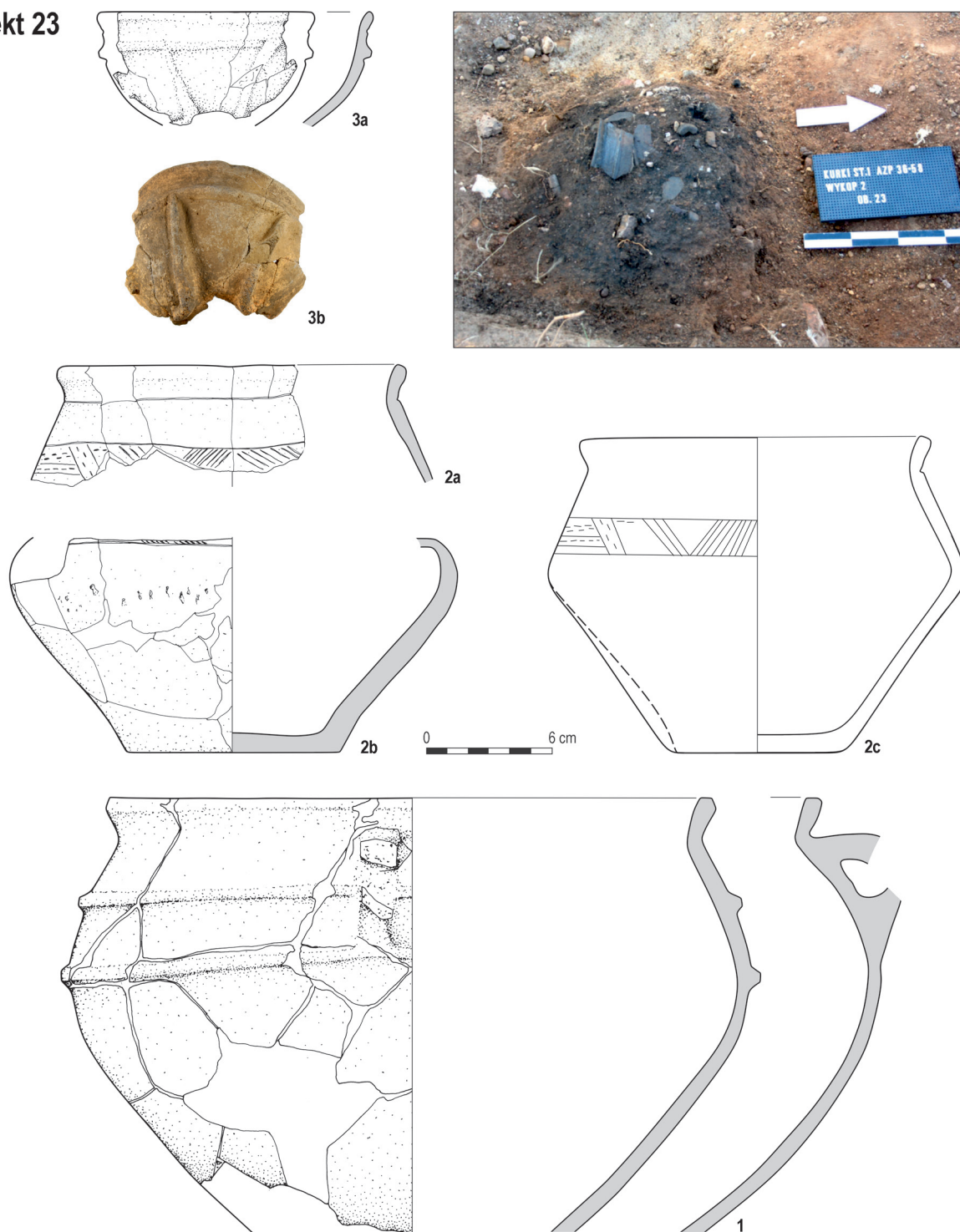
Ryc. 10. Kurki, pow. działdowski, stan. III. Obiekt 23: 1–3 – glina. Rys.: A. Czubińska (1–3a), M. Woźniak (2c).
