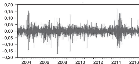
Rys. 5. Zmienność czasowa stóp zwrotu spot dla ropy crude WTI w badanej próbie. Źródło: badania własne.
