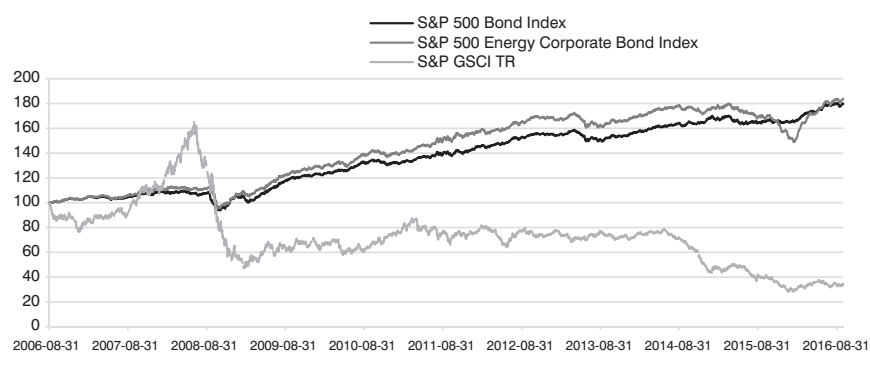
Rys. 4. Kształtowanie się poziomu indeksów rynku obligacji i obligacji korporacyjnych na tle zmian indeksu rynku surowcowego. Źródło: S&P Dow Jones Indices.
