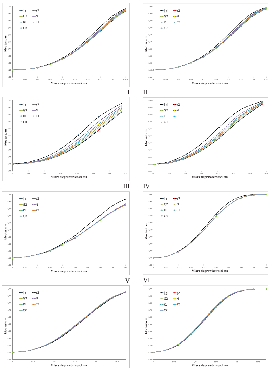
Rysunek 3. Moc testów niezależności dla TD 2 \times 4 oraz liczebności próby n I. Schemat A, n = 150 V. Schemat C, n = 50 II. Schemat A, n = 175 VI. Schemat C, n = 100 III. Schemat B, n = 150 VII. Schemat D, n = 30 IV. Schemat B, n = 200 VIII. Schemat D, n = 50
