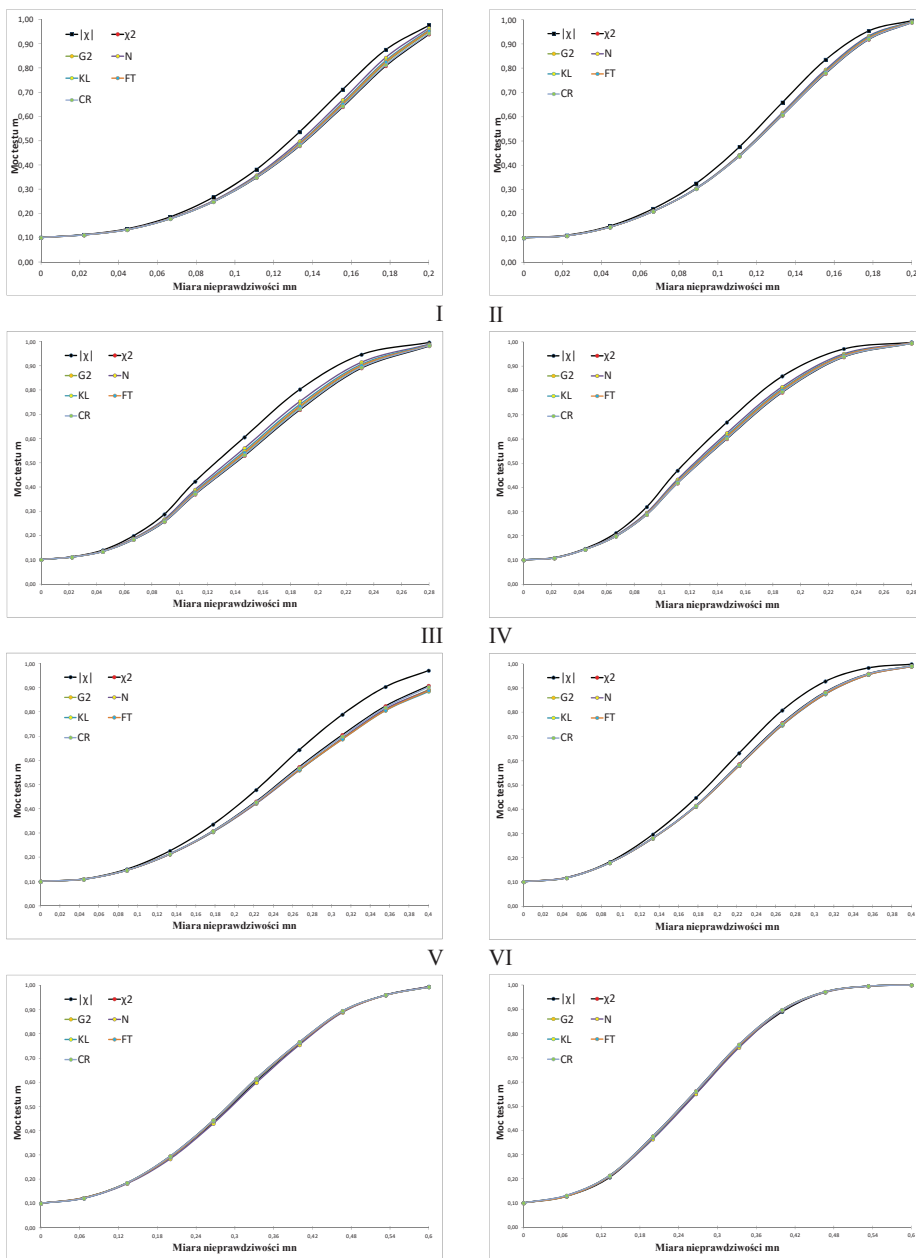
Rysunek 2. Moc testów niezależności dla TD 2 \times 3 oraz liczebności próby n I. Schemat A, n = 125 II. Schemat A, n = 150 III. Schemat B, n = 125 IV. Schemat B, n = 150 V. Schemat C, n = 50 VI. Schemat C, n = 75 VII. Schemat D, n = 30 VIII. Schemat D, n = 40
