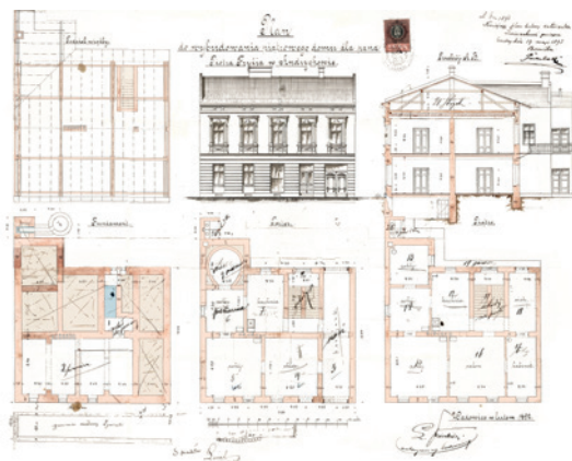
Plan murowanego domu nr 9 Piotra Frysia wykonany przez autoryzowanego budowniczego z Wadowic w lutym 1892 r. Źródło: ze zbiorów rodzinnych
