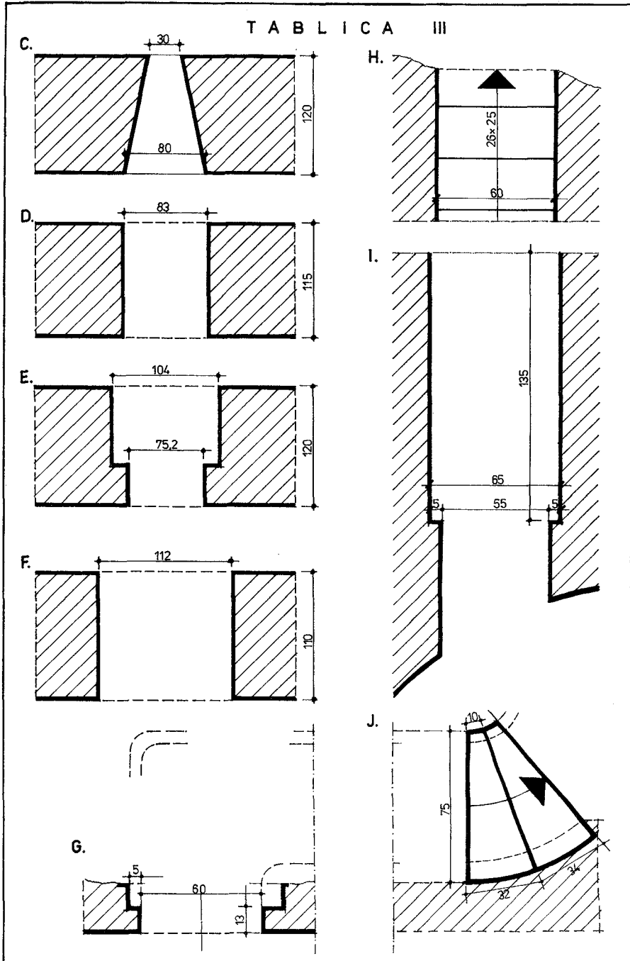
Tablica III. Ostrow Lednicki — wymiary otworów drzwiowych i okiennych — konstrukcje schodów
