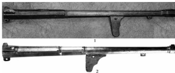
Fig. 2. 1- hakownica z zamku Chropyně; Dolínek 2004: Fig. 13; 2- hakownica z Kopenhagi; McLachlan 2010: 58
