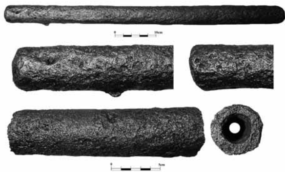
Fig. 9. Chełm, Plac E. Łuczковского. Hakownica nr inw. CH-Ł/110W/09. Fot. P. Strzyż
