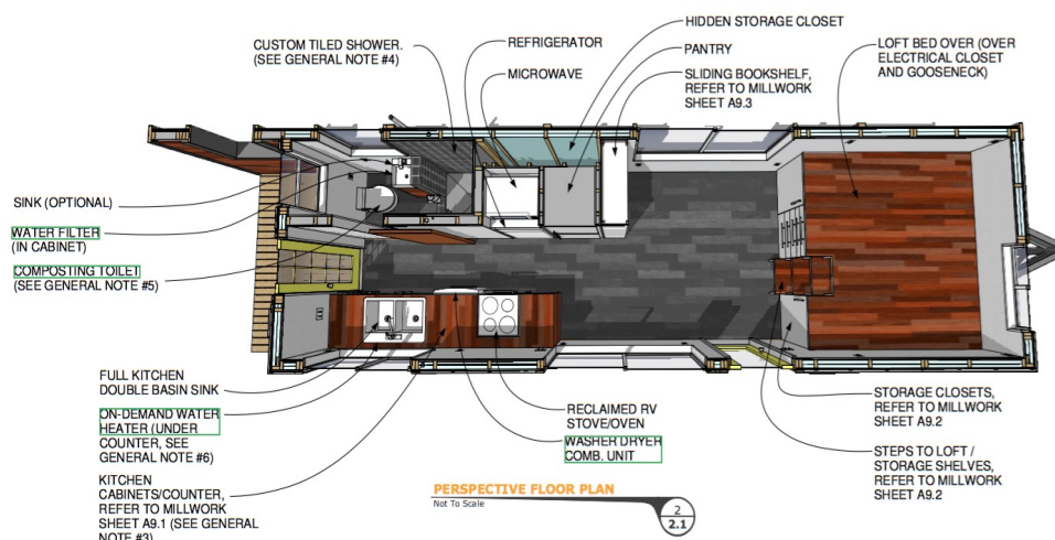
Fotografia 13. Macy Miller House, rzut.
