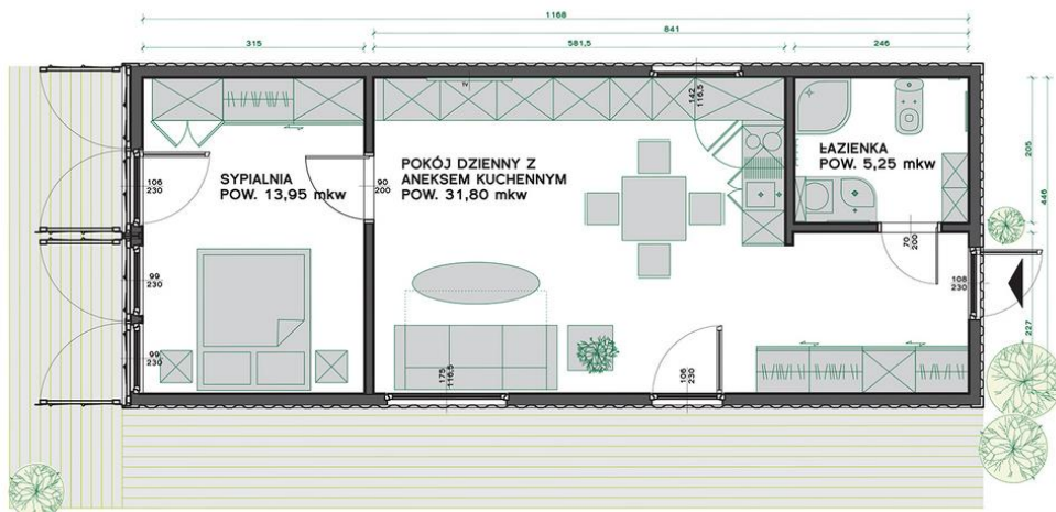
Fotografia 15. Polski dom z kontenera, przykładowy rzut.
