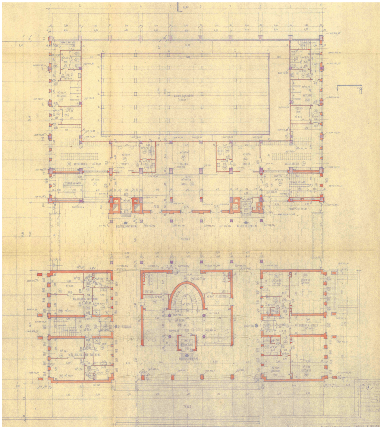
Il. 4. J. Krug, projekt KS Włóknarz, 1951. Rzut parteru (źródło: ANK, ABM 29/789/1128)
