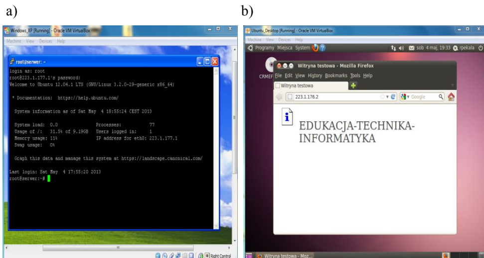
Rys. 4. Połączenia od aplikacji klienckich do serwerowych: a) połączenie ze stacji Windows XP za pomocą klienta ssh (putty.exe) do stacji Ubuntu_serwer, b) połączenie z przeglądarki stacji Ubuntu_desktop do serwera witryn na stacji Windows_serwer
