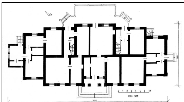
Rys. 2. Plan zabytkowego budynku dworskiego w Prusinowicach Źródło: S. Małyżko, Karta ewidencyjna zabytków architektury i budownictwa , Ośrodek Dokumentacji Zabytków w Warszawie, 1997
