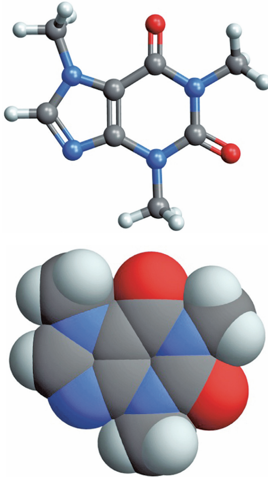
Ryc. 1, 2. Dwa pogładowe modele cząsteczki kofeiny C_8H_{10}N_4O_2 (rysunki wykonano korzystając z programu Mathematica firmy Wolfram Research)
